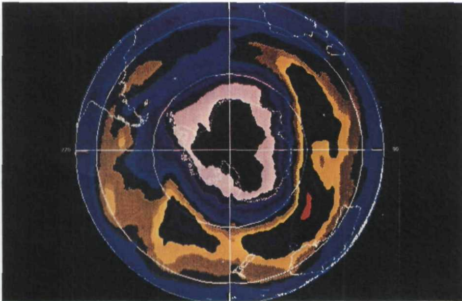
3 - الفجوة التي حدثت في طبقة الاوزون، الواقية من الاشعة الضارة في منطقة القطب الجنوبي، كما اوضحتها وسائل الرصد والتحليل بالافمار الصناعية.
