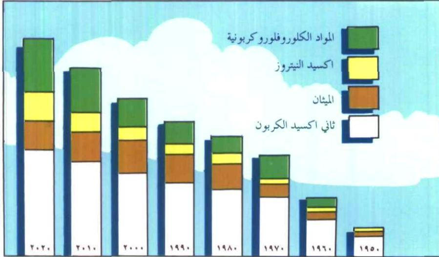
٢ - نسب الغازات الصوبية في الغلاف الجوي والزيادة المتوقعة ان تضرراً عليها اذا لم تتخذ الاجراءات اللازمة للحد من انتشارها.
