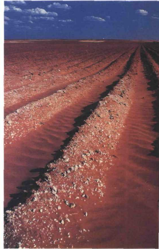
٧ - اراض زراعية لحق بها التصحر نتيجة للجفاف .
